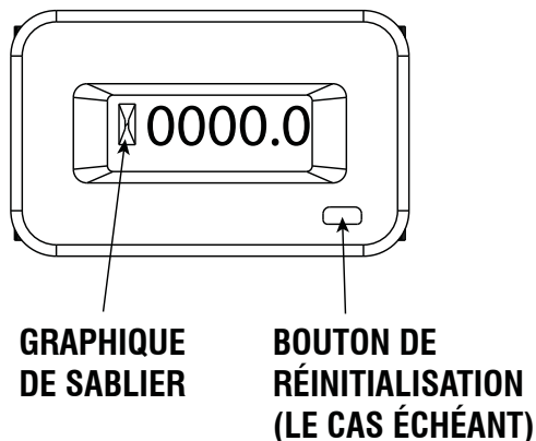
Figure 7 - Horomètre
