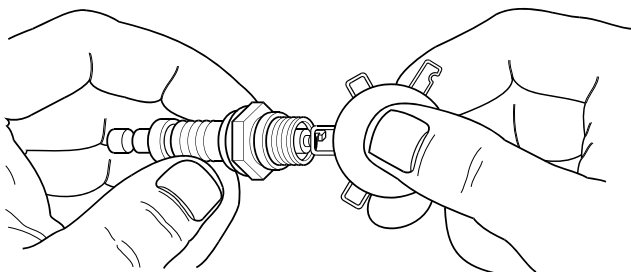
Schéma 14 - Écartement de la bougie d'allumage
