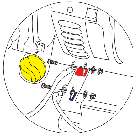
Schéma 15 - Branchements de la batterie
